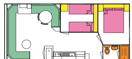
8,77 X 4m 2-bed douche en toilet
